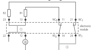
F227 - module wiring diagram
