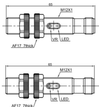
Emitter
