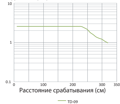
Обнаружение прозрачных объектов (PSS/PSM-GM2...R/-E2)
