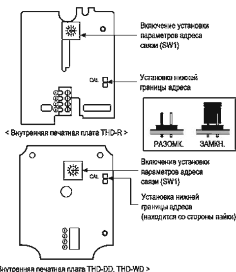
< Внутренняя печатная плата THD-DD, THD-WD >
